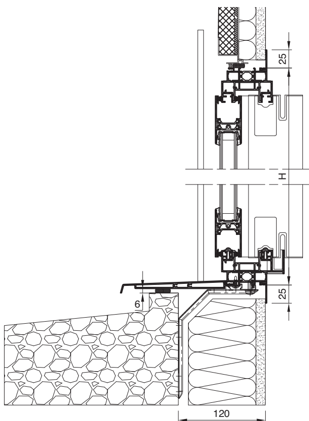
Sur maçonnerie
